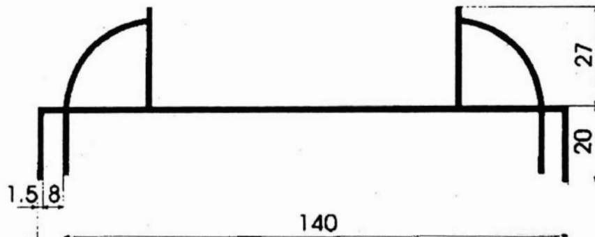
Profil No. 6240 1.360 Kg/m
