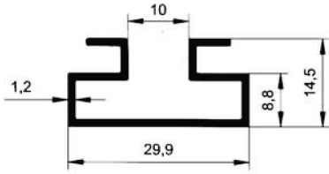
5519 0.277 kg/m
