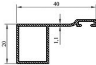
Profil N o : 2507 Ag ırık : 0,295 kg/m
