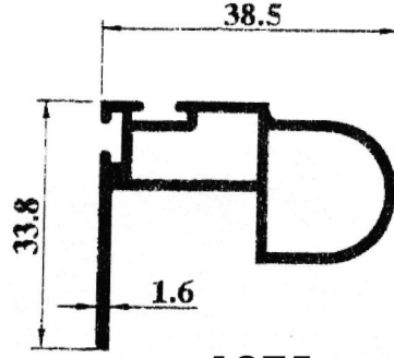
1275 0,520 kg/m
