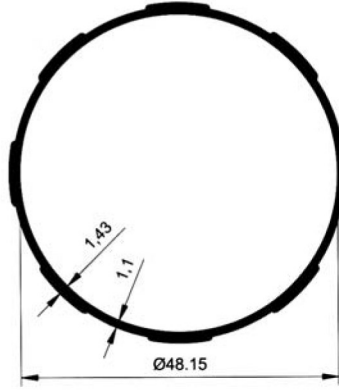
5449 0.531 kg/m
