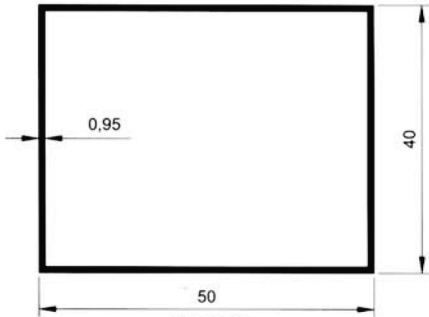
5103 0.453 kg/m
