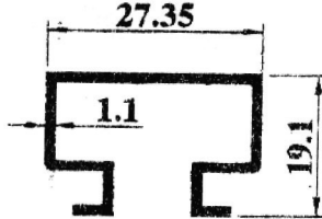
1278 0,254 kg/m
