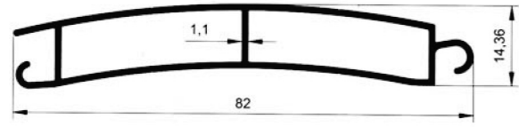
5611 0.577 kg/m
