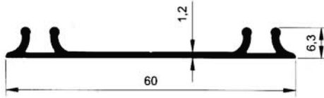
5522 0.282 kg/m
