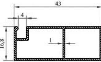
Profil N o : 2505 Ag ırık : 0,373 kg/m
