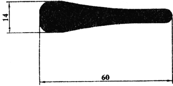
1296 (1.416 Kg/m)
