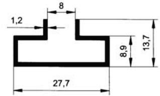
5524 0.228 kg/m
