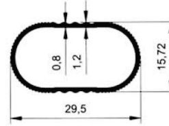
5812 0.198 kg/m
