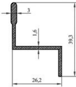
Profil N o : 2510 Ag ırık : 0,317 kg/m
