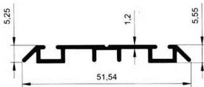
5810 0.281 kg/m
