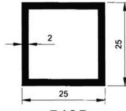
5485 0.499 kg/m
