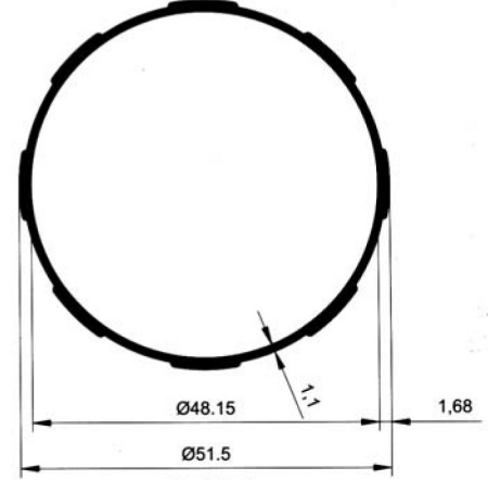
5434 0.580 kg/m
