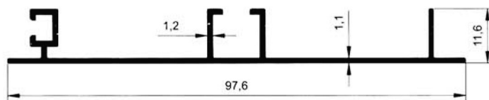
5659 BAZA 0.473 kg/m
