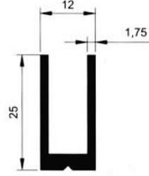
5076 0.315 kg/m
