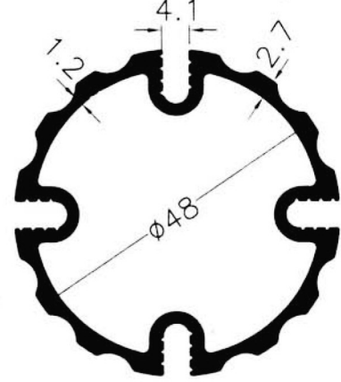
5272 0.983 Kg/m
