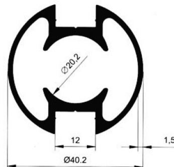
5638 0.883 kg/m
