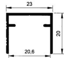
5548 0.214 kg/m
