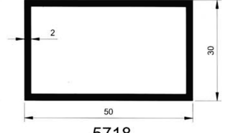
5718 0.823 kg/m
