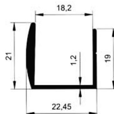
5808 0.247 kg/m
