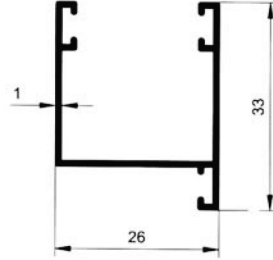
5123 0.274 kg/m
