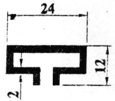
1280 0,325 kg/m
