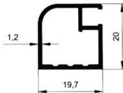
5811 0.265 kg/m
