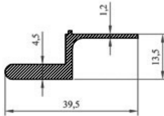
Profil N o : 2511 Ag ırık : 0,358 kg/m
