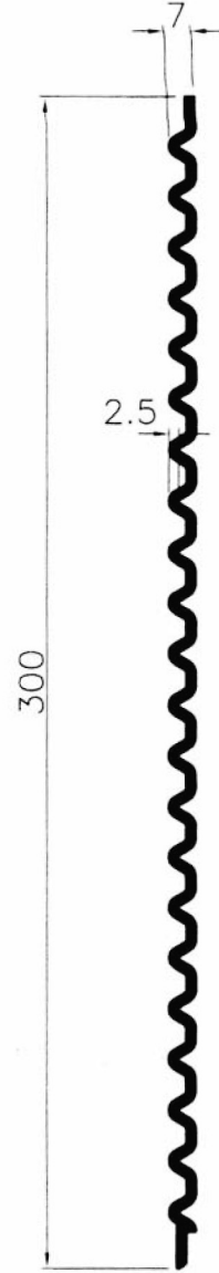
4649 2.674 Kg/m Ölçek: 1/2
