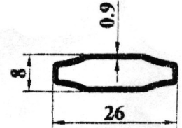
1284 0,170 kg/m
