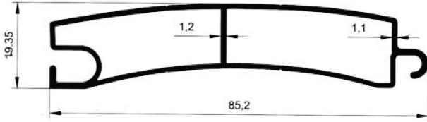
5610 0.656 kg/m
