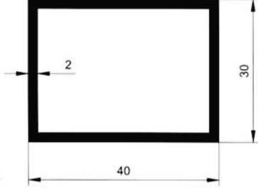
5720 0.715 kg/m
