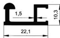
5564 0.230 kg/m
