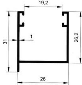
5122 0.256 kg/m
