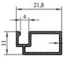
Profil N o : 2504 Ag ırık : 0,179 kg/m
