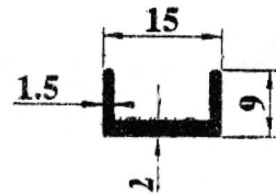
1286 0,140 kg/m
