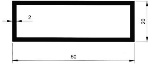
5484 0.821 kg/m
