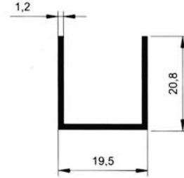
5090 0.189 kg/m
