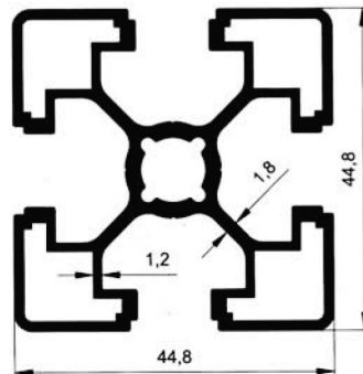
5631 1.299 kg/m
