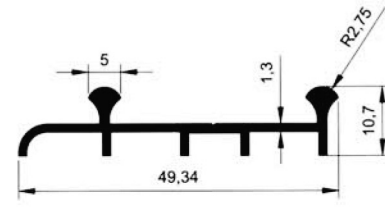
5809 0.318 kg/m
