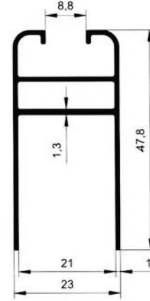
5803 0.427 kg/m
