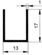
5120 0.122 kg/m
