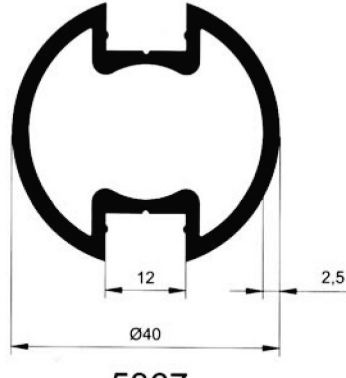
5367 0.951 kg/m
