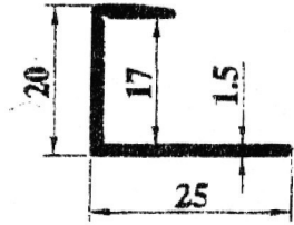
1281 0,200 kg/m
