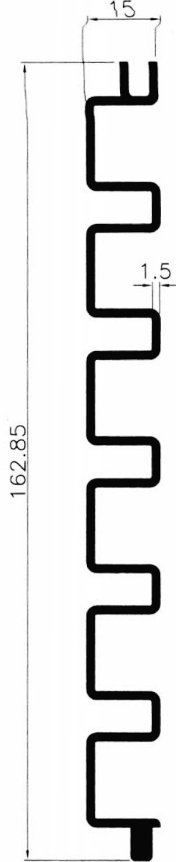
3378 1.345 Kg/m
