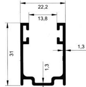
5752 0.383 kg/m
