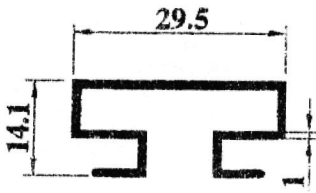
1277 0,230 kg/m
