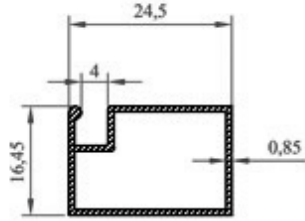
Profil N o : 2501 Ag ırık : 0,198 kg/m
