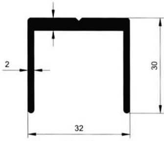
5074 0.622 kg/m
