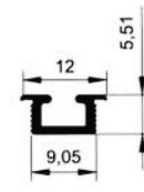
5813 0.070 kg/m
