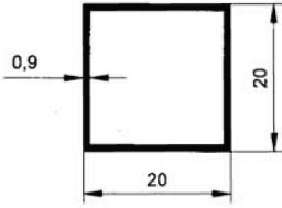
5603 0.185 kg/m
