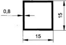
5604 0.122 kg/m
