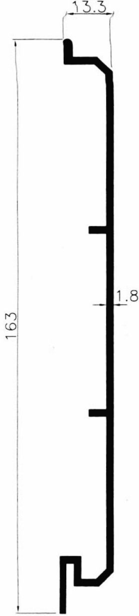
1640 0.998 Kg/m
