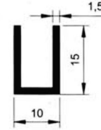
5389 0.151 kg/m
