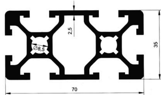
5411 2.233 kg/m
