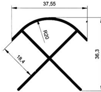
5534 0.409 kg/m
