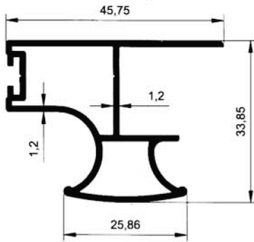
5529 0.585 kg/m
