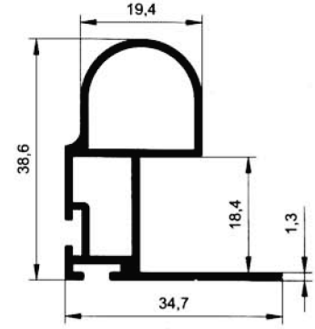
5521 0.509 kg/m
