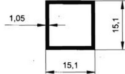
1037 0.160 kg/m
