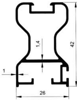
5804 0.495 kg/m
