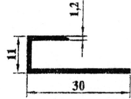
1276 0.165 kg/m
