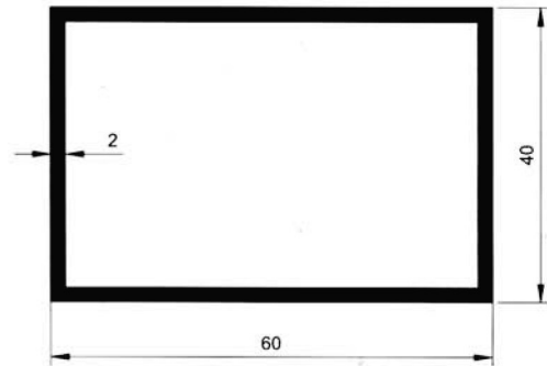
5489 1.038 kg/m
