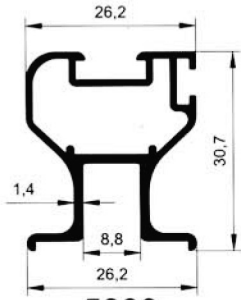
5800 0.436 kg/m
