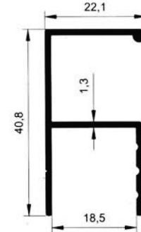
5806 0.391 kg/m
