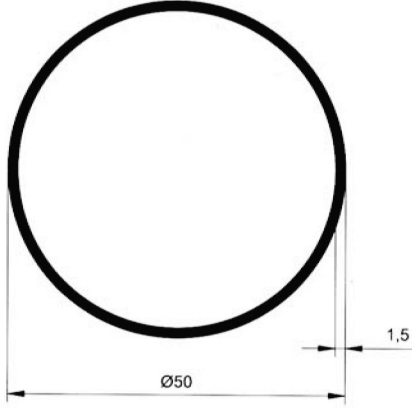
5361 0.619 kg/m
