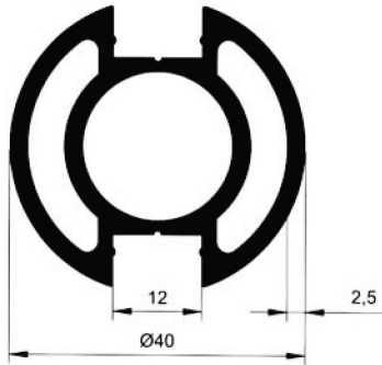
5369 1.249 kg/m
