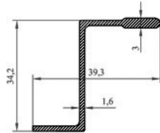
Profil N o : 2509 Ag ırık : 0,355 kg/m
