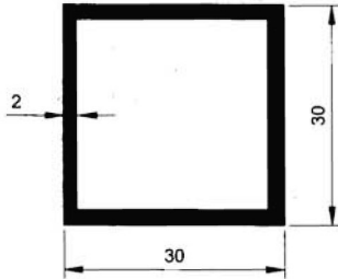
5486 0.607 kg/m
