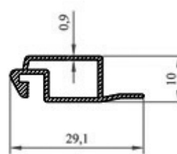
Profil N o : 2512 Ag ırık : 0,180 kg/m
