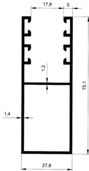
5621 0.918 kg/m
