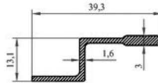
Profil N o : 2508 Ag ırık : 0,256 kg/m
