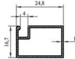
Profil N o : 2502 Ag ırık : 0,235 kg/m
