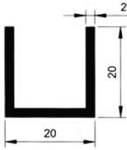
5402 0.303 kg/m
