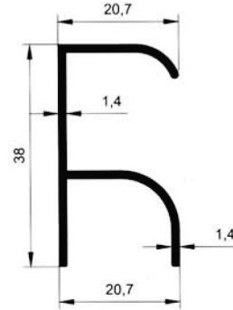
5802 0.338 kg/m
