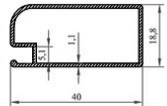
Profil N o : 2513 Ag ırık : 0,347 kg/m
