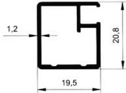
5801 0.268 kg/m
