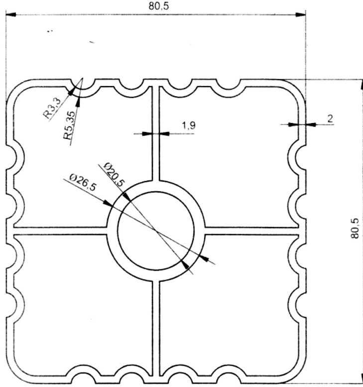
2040 2,972 kg/m
