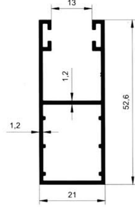
5749 0.542 kg/m
