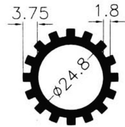
3836 0.460 Kg/m
