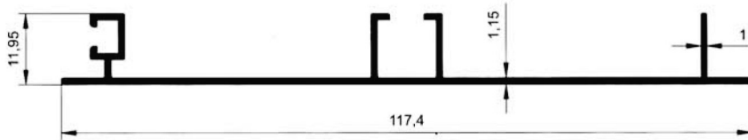
5657 BAZA 0.540 kg/m
