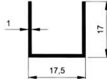
5121 0.134 kg/m
