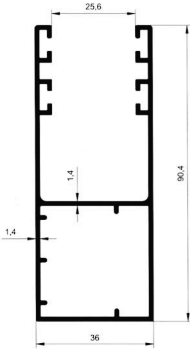
5750 1.166 kg/m
