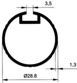
5609 0.349 kg/m
