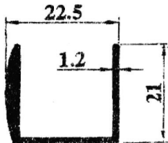
1285 0,250 kg/m
