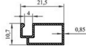
Profil N o : 2503 Ag ırık : 0,152 kg/m
