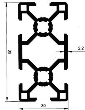
5776 1.525 kg/m
