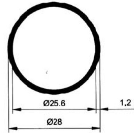
5724 0.262 kg/m
