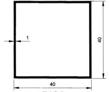
5104 0.422 kg/m
