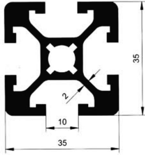
5354 0.1334 kg/m
