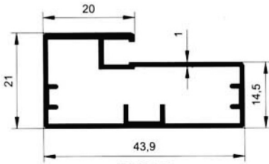
5807 0.443 kg/m
