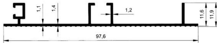
5658 BAZA 0.502 kg/m
