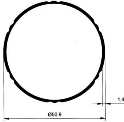
5608 0.556 kg/m
