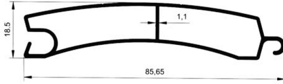
5394 0.653 kg/m
