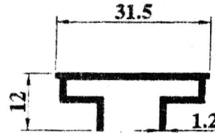
1279 0,223 kg/m
