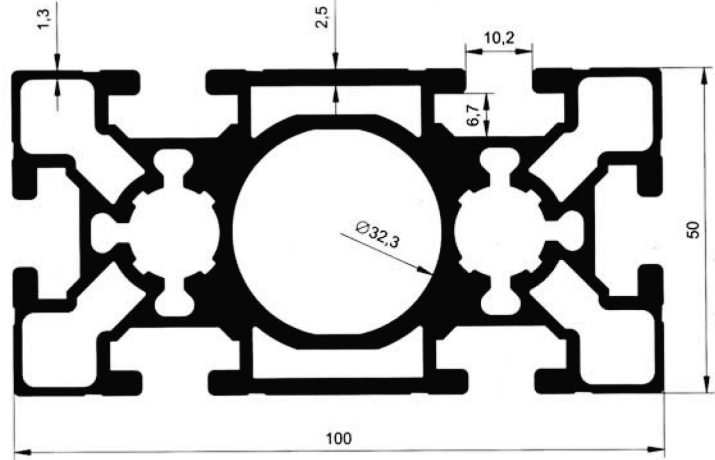
5518 4.387 kg/m
