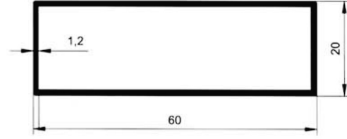
5587 0.500 kg/m
