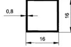
5732 0.132 kg/m
