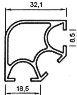
1227 Dikme 0.605 kg/m.
