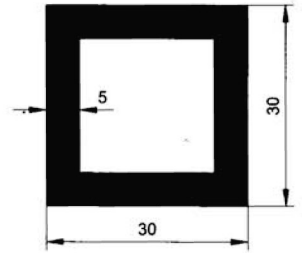
5705 1.355 kg/m
