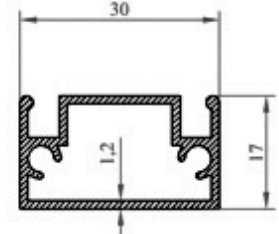
Profil N o : 5138 Ag ırık : 0,369 kg/m
