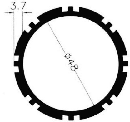
3835 1.147 Kg/m
