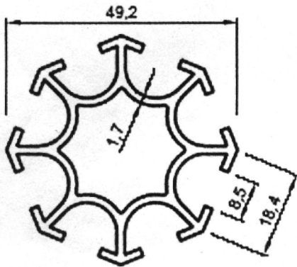
1225 Dikme 1.100 kg/m.
