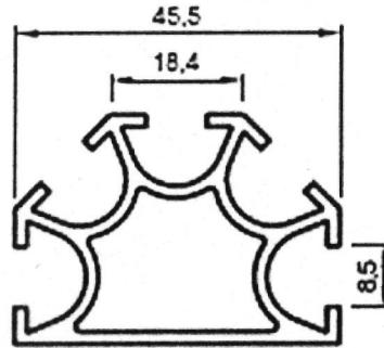
1226 Dikme 0.900 kg/m.
