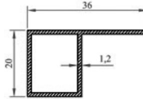
Profil N o : 2506 Ag ırık : 0,284 kg/m
