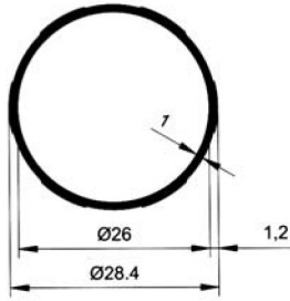
5433 0.252 kg/m
