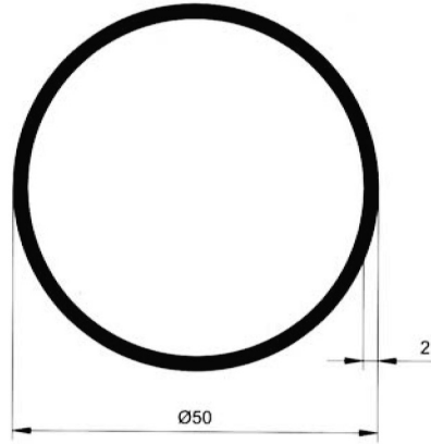
5362 0.817 kg/m
