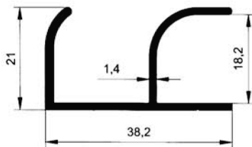
5559 0.357 kg/m
