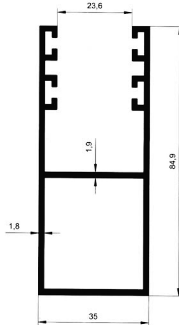
5622 1.389 kg/m
